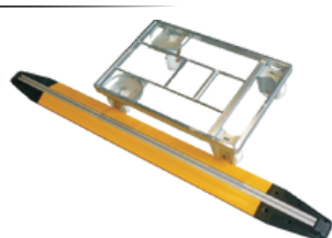
Affiancare le ruote del carrello al binario
